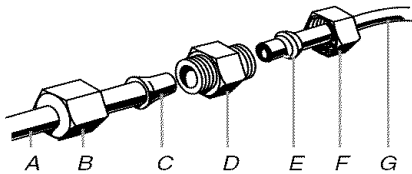
A. Tubería de agua del refrigerador D. Acoplamiento (adquirido) B. Tuerca (provista) E. Fécula (adquirida) C. Bulbo F. Tuerca (adquirida) G. Línea de agua de la casa
