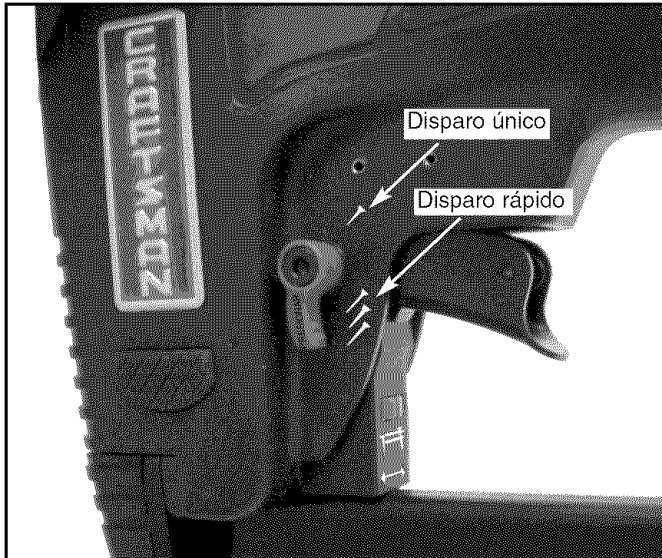
Figura 5 – Presione y Gire el Interruptor para Seleccionar el Modo de Operación
