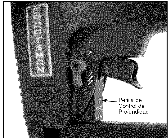
Figura 6 – Ajuste del Control de Profundidad
