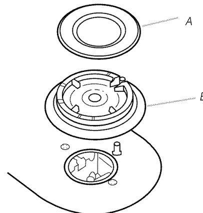
A. Tapa del quemador B. Quemador
