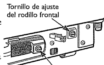
Tornillo ajustable del rodillo trasero (solamente en modelos de estilo empotrado) Use este tornillo si el refrigerador tiene uno
