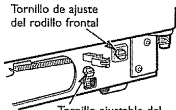
Tornillo ajustable del rodillo trasero (solamente en modelos de estilo empotrado) Use este tornillo si el refrigerador no tiene el tornillo que se muestra arriba.
