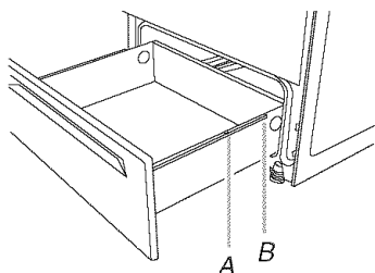
A. Encoche de la butée de tiroir B. Extrémité du rail latéral
