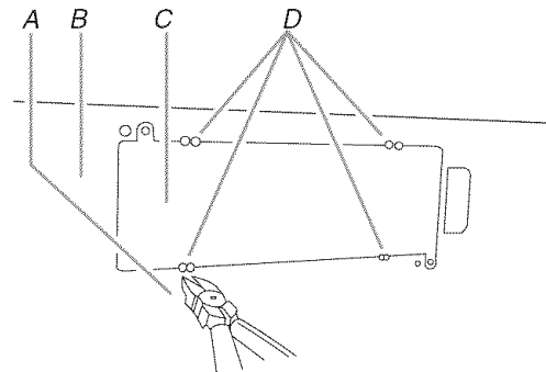
A. Pince coupante B. Arrière du four à micro-ondes C. Couvercle de fermeture de la bouche de sortie D. Points de fixation
