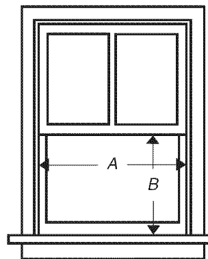
A. 27" mín. (68,6 cm) B. 16 \frac{1}{4} " mín. (41,3 cm)
