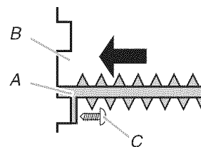
A. Cortina lateral contra la ranura de la ventana B. Ranura de la ventana C. Tornillo de cabeza redonda #8 x \frac{3}{4} "
