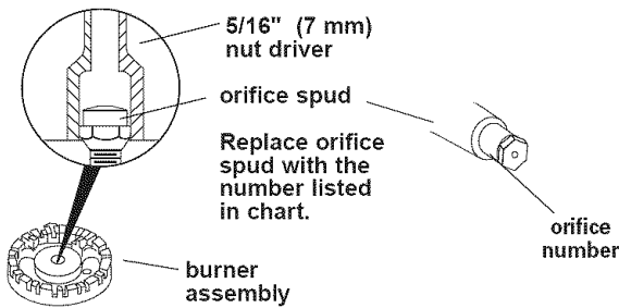
Natural gas orifice spud
