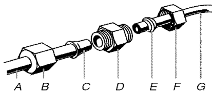
A. Tubería de agua al refrigerador E. Férula (adquirida) B. Tuerca (provista) F. Tuerca (adquirida) C. Bulbo G. Línea de agua de la casa D. Acoplamiento (provisto)
