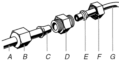
A. Canalisation d'arrivée d'eau du réfrigérateur E. Virole (à acheter) B. Écrou (fourni) F. Écrou (à acheter) C. Renflement G. Canalisation d'eau du domicile D. Raccord (fourni)
