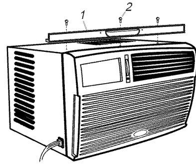
1. Canal superior 2. Tornillo de cabeza de cono achatado #10 x 3/8 pulg.
