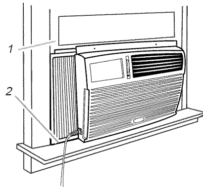
1. Marco de la ventana 2. Riel inferior detrás del lado posterior del obturador de la ventana
