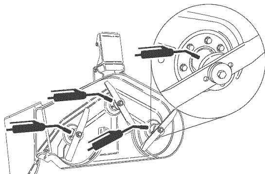
Figura 16. Lubricación del Árbol de Sujeción
