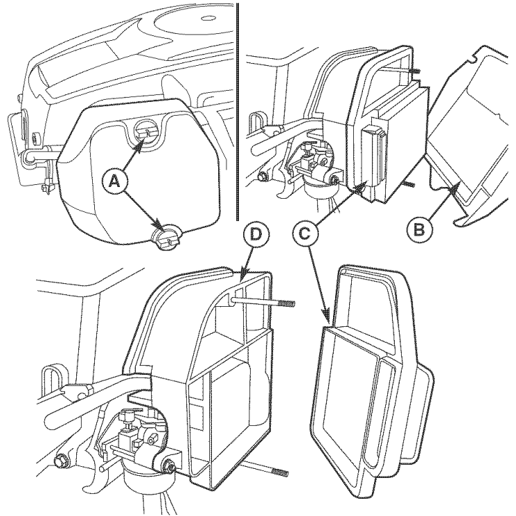
Figura 28. Ensamblaje del filtro de aceite - Modelos Kohler A. Botón de la cubierta del filtro de aire B. Cubierta C. Filtro de aire D. Base
