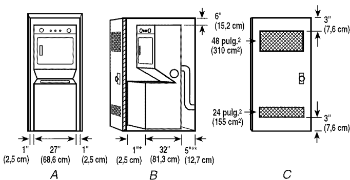
A. Lugar empotrado B. Vista lateral - clóset o lugar confinado C. Puerta del clóset con orificios de ventilación
