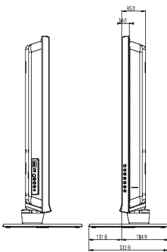
VISTA LATERAL
