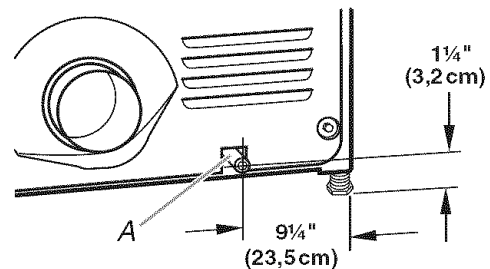
A. Tuyau NPT de la sécheuse de 3/8"
