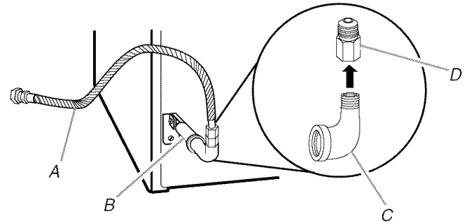
A. Connecteur à gaz souple de 3/8"
