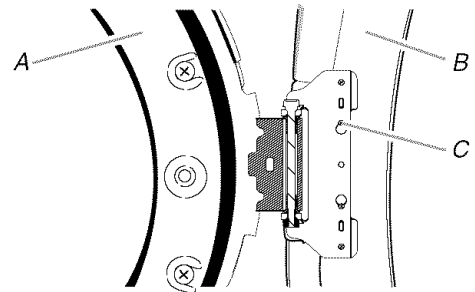
A. Porte de la sècheuse B. Sècheuse C. Insérer cette vis en premier.
