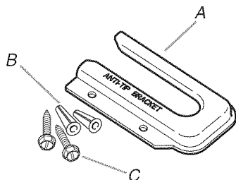
A. Bride antibasculement B. Chevilles de plastique (2) C. Vis n°10 x ½" (2)
