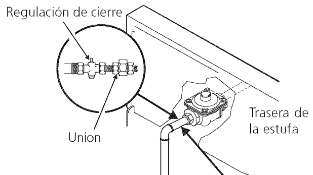
Acoplamiento de conector flexible Figura 5
