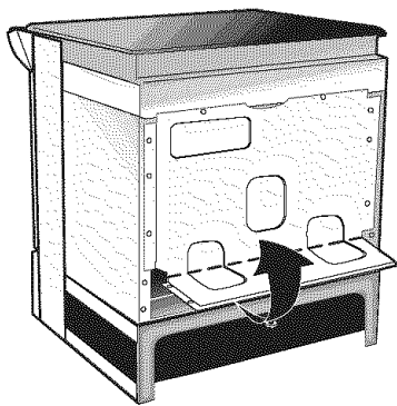
RECOURBEZ ICI LE COUVERCLE ARRIÈRE POUR ACCÉDER AU RACCORDEMENT ÉLECTRIQUE Figure 3
