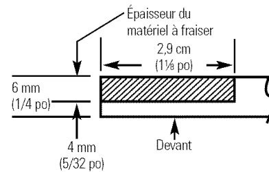
Exemple de fraisage
