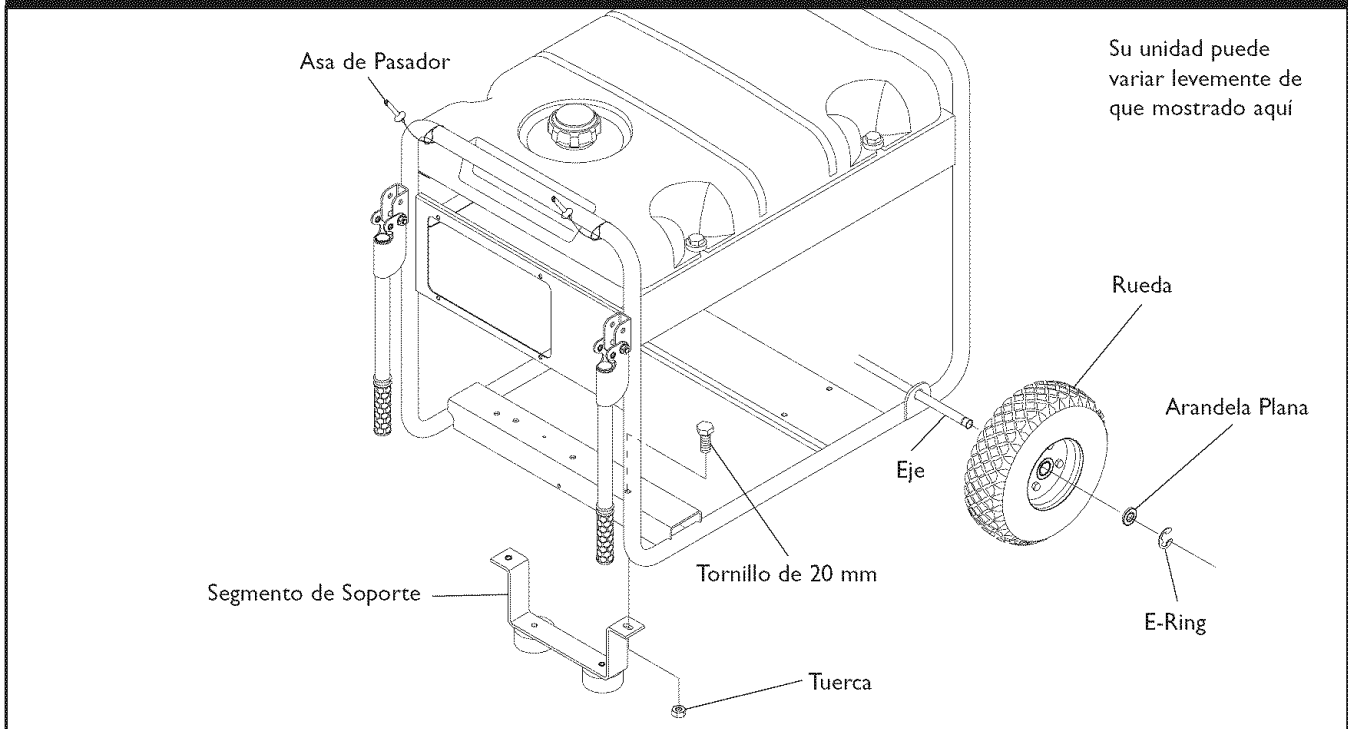
Figura 13 — Instale el Juego de Ruedas
