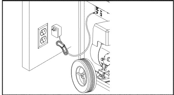
Figura 22 — Enchufe Hembra del Cargador de Flotación
