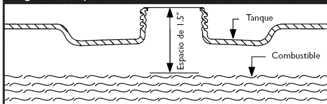
Figura 15 - Espacio de Combustible
