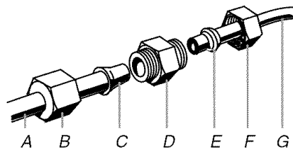
A. Conduit vers le réfrigérateur B. Écrou (fourni) C. Renflement D. Raccord (fourni) E. Virole (à acheter) F. Écrou (à acheter) G. Canalisation d'eau du domicile
