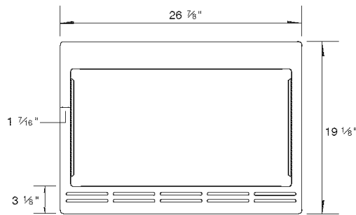
Bâti d'encastrement 27"
