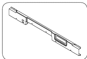
Ménsula superior
