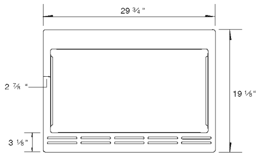
Bâti d'encastrement 30"
