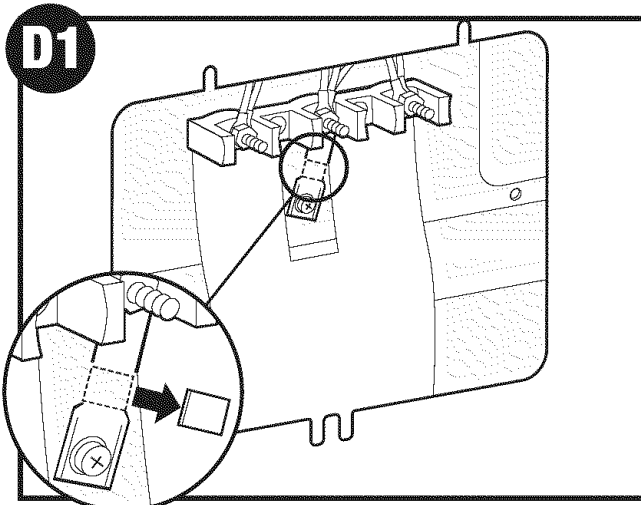
D1 Part of copper ground strap MUST be cut out and removed./Une partie de la bande en cuivre de mise à la terre DOIT être coupée et enlevée./Una parte o la totalidad de la cinta de conexión a tierra DEBE ser cortada y descartada.
