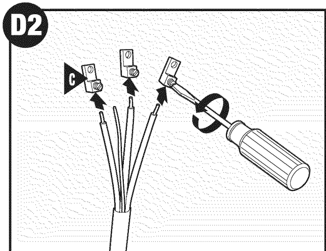
D2 Attach lugs. See Torque specifications./Fixez les oreilles de fixation. Voyez les spécifications de serrage./Fije las tuercas. Consulte las especificaciones del torque.
