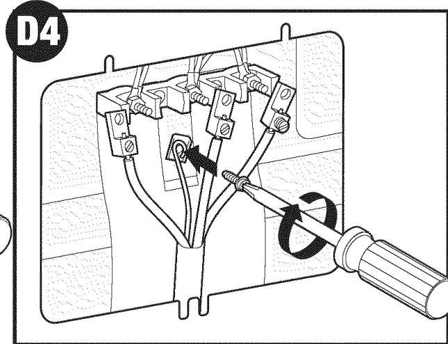
D4 Connect ground wire./Raccordez le fil de mise à la terre./Conecte el alambre de tierra.
