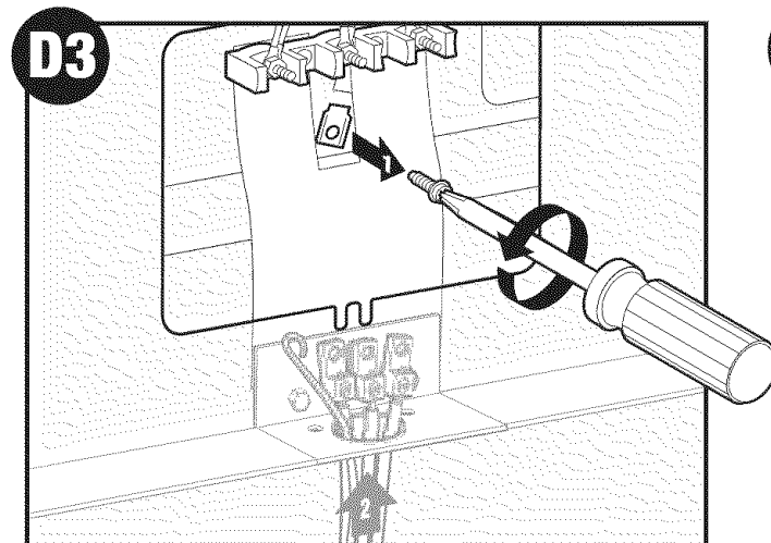
D3 Remove grounding screw, pull conduit through./Retirez la vis de mise à la terre, passez le conduit./Retire el tornillo de puesta a tierra y tire del conducto a través del agujero.
