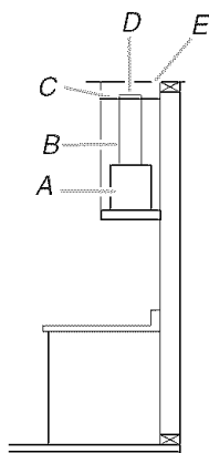
A. Hotte B. Système de décharge C. Sommet du placard D. Couvercle d'évent E. Plafond ou soffite
