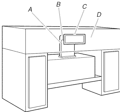
A. Conduit de 3/4" x 10" (8,3 cm x 25 cm) B. Coude 3/4" x 10" (8,3 cm x 25 cm) C. Couvercle d'évent D. Soffite
