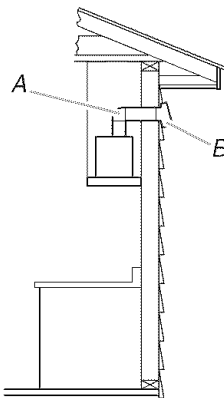
A. Conduit de 3/4" x 10" (8,3 cm x 25 cm) à travers le mur B. Bouche de décharge murale
