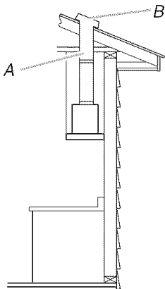
A. Conduit de 3/4" x 10" (8,3 cm x 25 cm) à travers le toit B. Bouche de décharge sur toit
