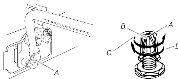
A. Gicleur B. Broche C. Gaz naturel : augmentation du débit de gaz - augmentation de la taille des flammes (préréglage à l'usine pour gaz naturel) D. Propane : réduction du débit de gaz - réduction de la taille des flammes
