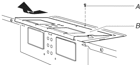
A. Vis B. Plaque de support du clapet
