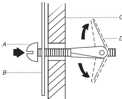
A. Vis 1/4-20 x 3" B. Plaque de montage C. Panneau de gypse D. Écrou articulé
