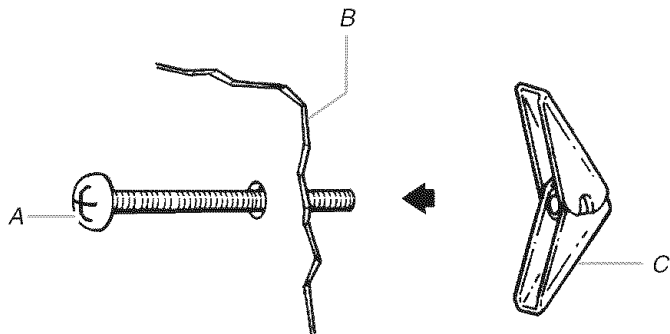
A. Vis 1/4-20 x 3" B. Plaque de montage C. Écrou articulé
