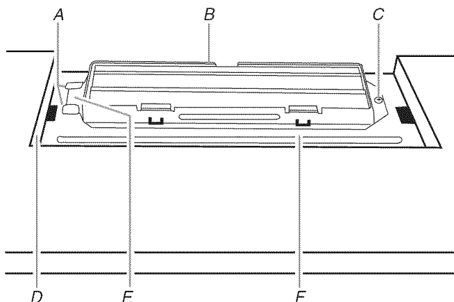
A. Pattes relevées B. Module du clapet anti-reflux C. Vis de tôlerie D. Ouverture découpée dans le placard mural E. Patte longue F. Plaque de support du clapet
