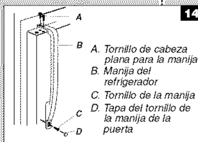
Frente del tornillo sellador de la manija de la puerta
