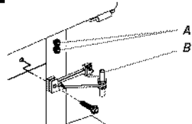
A. Vis de charnière à tête hexagonale de 7/16" B. Charnière centrale
