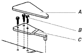
A. Tapa de la bisagra superior B. Tornillos de cabeza hexagonal para bisagra de 5/16" C. Bisagra superior
