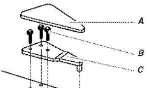
A. Couvercle de la charnière supérieure B. Vis de charnière à tête hexagonale de 7/16" C. Charnière supérieure
