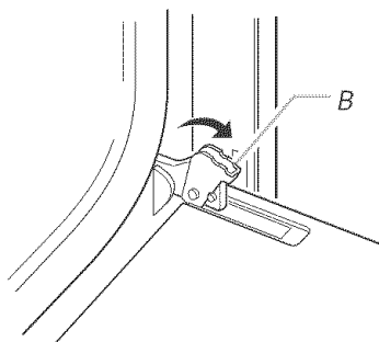
B. Porte du four - position de déverrouillage
