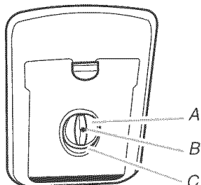
A. Bouchon pour l'agent de rinçage B. Témoin lumineux de l'agent de rinçage C. Distributeur d'agent de rinçage
