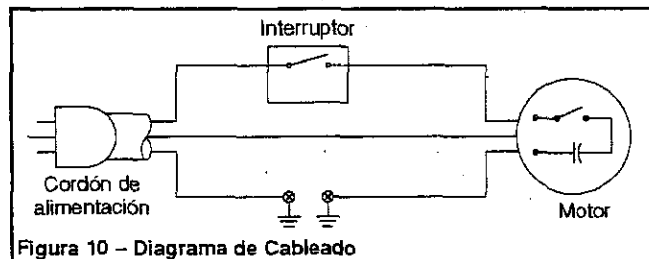
Figura 10 - Diagrama de Cableado
