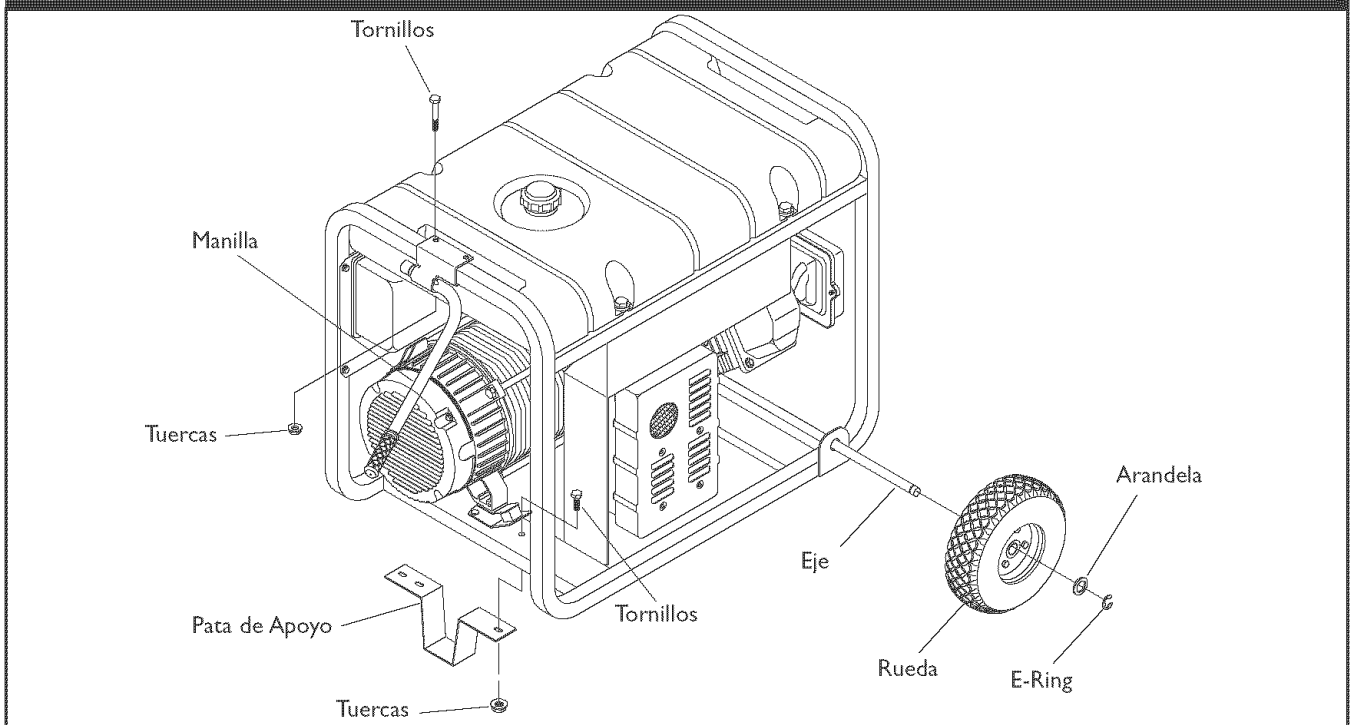
Figura 10 — Instale el Juego de Ruedas
