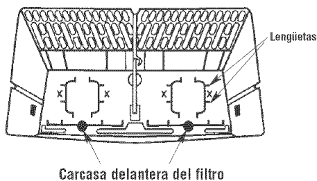
Parte delantera del humidificador Figura 5a. Las ubicaciones de los filtros están marcadas con una X
