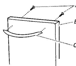
A. 2 tornillos insertados en los orificios desde el interior del cajón B. Parte superior del cajón C. Manija instalada en el frente del cajón
