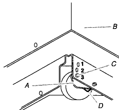
A. Conjunto de soporte de la rueda B. Gabinete del compactador C. Perno de localización D. Tornillo autorroscante (pivote)
