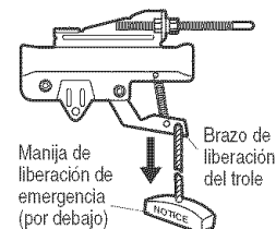
POSICIÓN DE DESENGANCHE MANUAL
