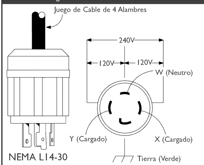
Figura 32 — 120/240 Volt AC, 30 Amp, Receptáculo de Seguridad
