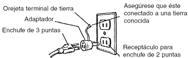
Figura 2 – Receptáculo con Adaptador para Enchufe de 2 Puntas
