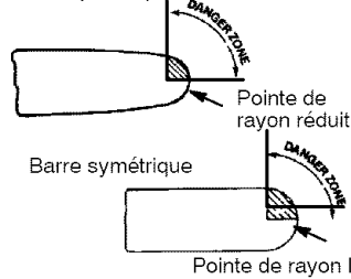
Barre symétrique au recul réduit
