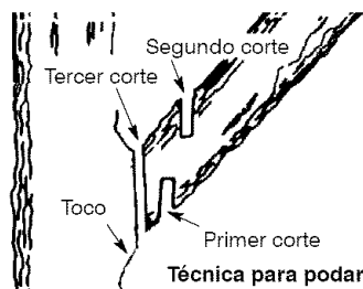
Técnica para podar
