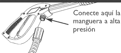
Figura 30 — Conecte la Manguera a alta Presión a la Pistola Rociadora
