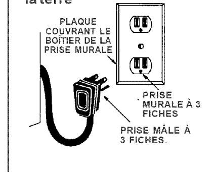
FIG. 11. Méthode recommandée de mise à la terre
