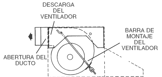
Descarga horizontal - posición del ventilador
