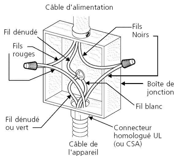
Figure 6 BOÎTE DE JONCTION À 3 FILS - MISE À LA TERRE
