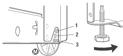
front leg pata delantera pied avant
