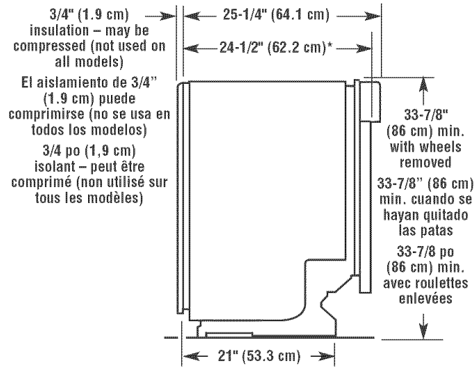
Side view Vista lateral Vue latérale
