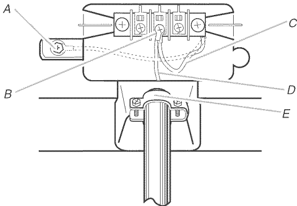
A. Tornillo conductor de tierra externo – La línea punteada ilustra la posición del hilo de tierra NEUTRO antes de moverlo al tornillo central de color plateado del bloque de terminal B. Tornillo central de color plateado del bloque de terminal C. Hilo neutro de puesta a tierra (verde con rayas amarillas) D. Hilo neutro (hilo blanco o central) E. Protector de cables de 3/4" (1,9 cm), que esté en la lista de UL
