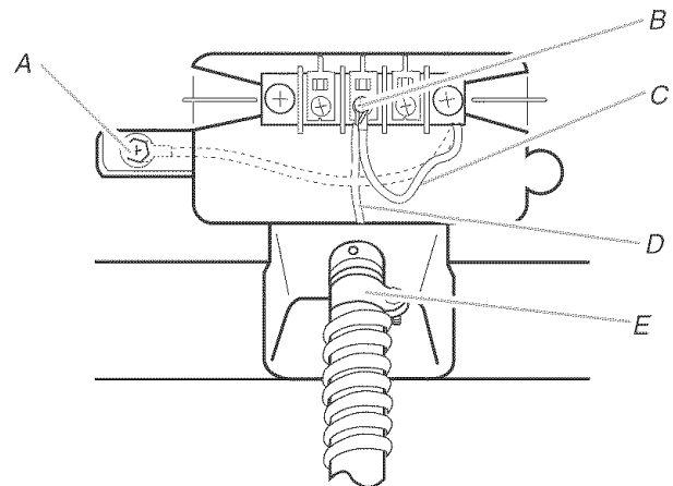
A. Tornillo conductor de tierra externo – La línea punteada ilustra la posición del hilo de tierra NEUTRO antes de moverlo al tornillo central de color plateado del bloque de terminal B. Tornillo central de color plateado del bloque de terminal C. Hilo neutro de puesta a tierra (verde con rayas amarillas) D. Hilo neutro (hilo blanco o central) E. Protector de cables que esté en la lista de UL de 3/4" (1,9 cm)
