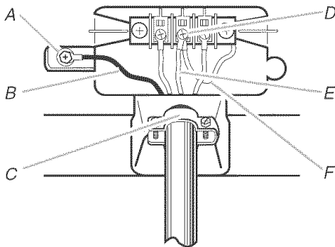
A. Tornillo conductor de tierra externo B. Hilo de tierra (verde o desnudo) del cable de suministro eléctrico C. Protector de cables que esté en la lista de UL de 3/4" (1,9 cm) D. Tornillo central de color plateado del bloque de terminal E. Hilo neutro (hilo blanco o central) F. Hilo neutro de puesta a tierra (verde con rayas amarillas)
