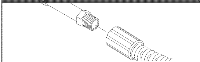
Figura 29 — Conectar la Manguera de Alta Presión a la Toma de Agua
