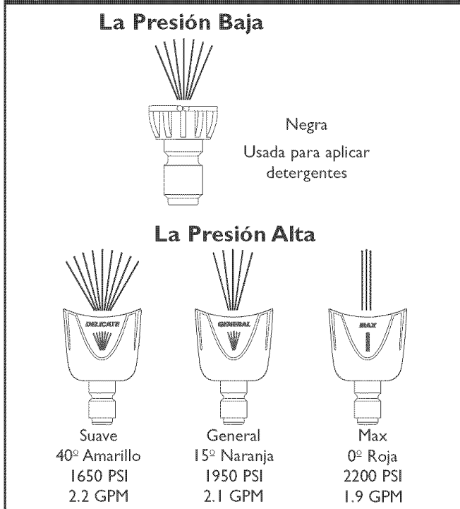
Figura 36 — Rocío los Modelos del Boquilla
