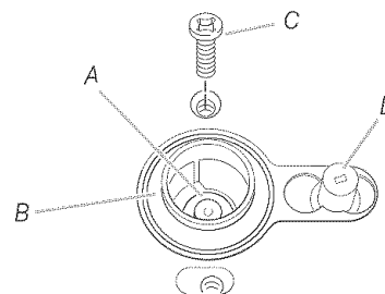
A. Gicleur B. Porte-gicleur C. Vis D. Électrode d'allumage
