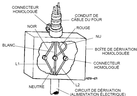
CUISINIÈRE RELIÉE À LA MASSE PAR LE CONDUCTEUR NEUTRE INSTALLATION À TROIS FILS
