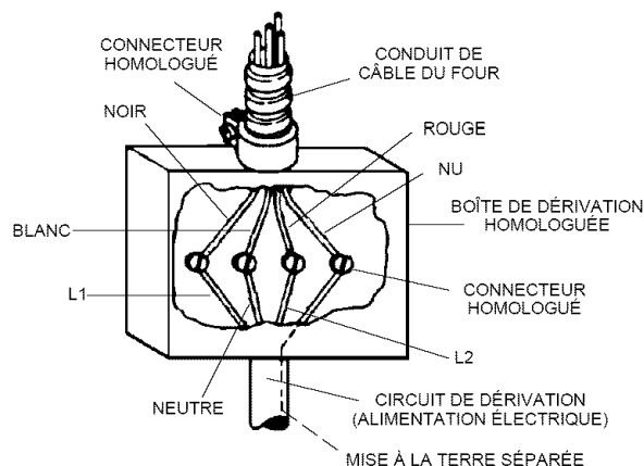
MÉTHODE DE CÂBLAGE SI LE CODE NE PERMET PAS LA MISE À LA MASSE PAR LE CONDUCTEUR NEUTRE, ÉGALEMENT REQUISE DANS LES MAISONS MOBILES.
