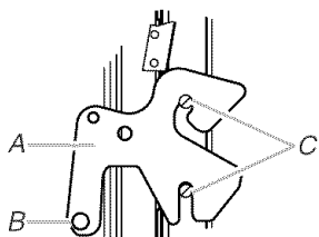
A. Ganchos de suspensión de las bisagras B. Bisagra del marco de la puerta C. Pernos de apoyo
