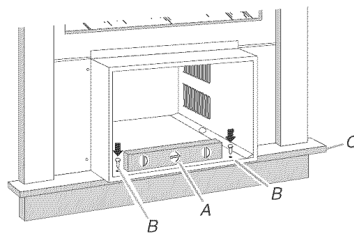
A. Nivel B. Tornillo para madera C. Umbral de la ventana
