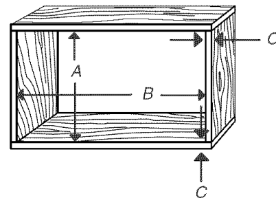
A. 19 3/4" (50,2 cm) C. Espesor de la madera B. 26 1/2" (66,1 cm)
