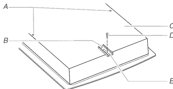
A. Trous de vis d'attache pour emplacement facultatif à l'avant et à l'arrière. B. Bride de fixation (emplacements aux extrémités recommandés) C. Partie inférieure de la boîte de brûleur D. Vis d'attache E. Emplacement (recommandé) de la vis d'attache
